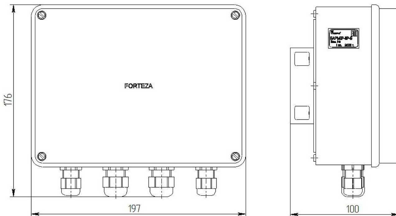
Рисунок 1 – Внешний вид коробки (стандартная комплектация)
